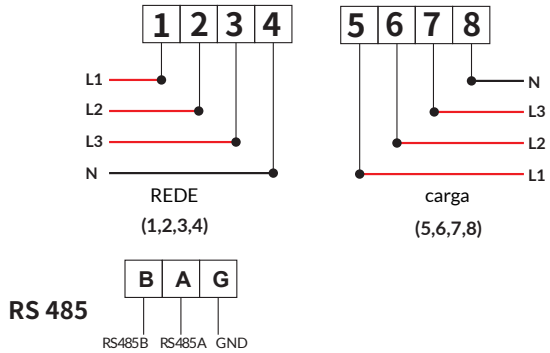
Figura 7.1 Medidor Eastron
