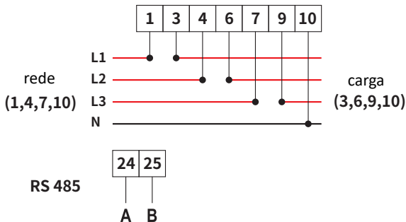
Figura 7.26 Medidor CHINT
