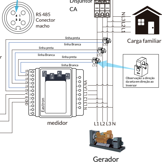
Figura 7.8 Diagrama de conexão do medidor Eastron
